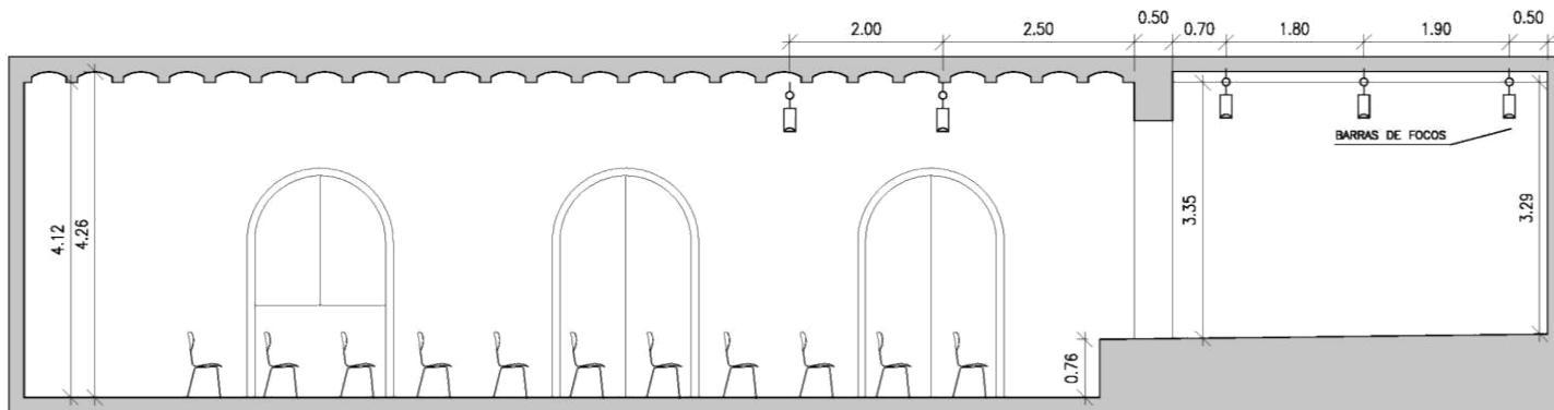
SECCIÓN LONGITUDINAL E/1:100
